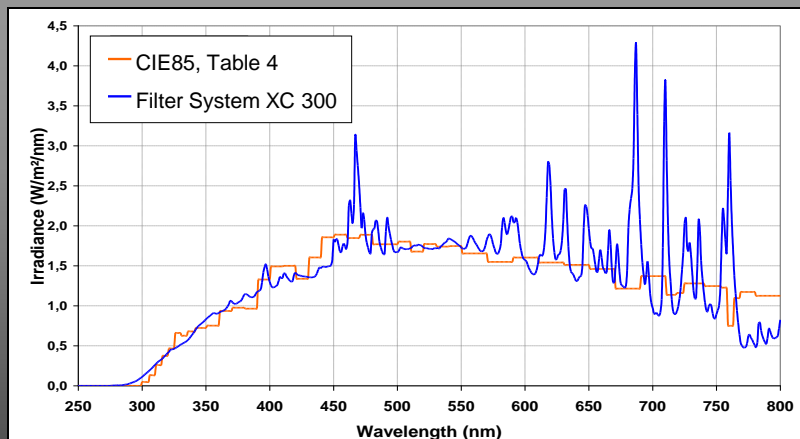
XENOCHROME® 300 для имитации условий на открытом воздухе (Транспорт/Хранение) -Daylight
