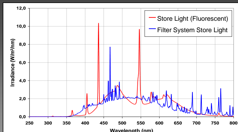
XENOCHROME® 300 плюс внешний цилиндр Store Light для имитации условий освещения в супермаркете (Хранение / Продажа)
