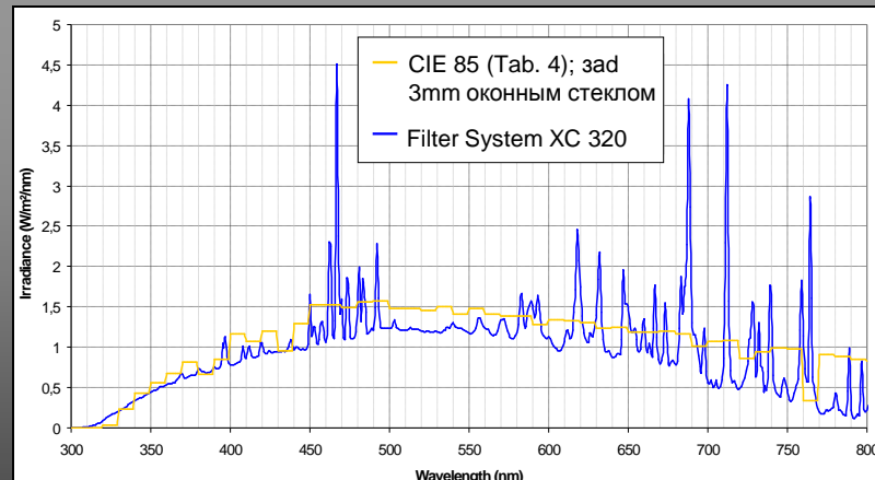
XENOCHROME® 320 для имитации условий за оконным стеклом внутри помещения (Хранение / Продажа / Потребление)
